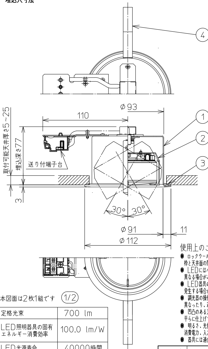
埋込穴寸法
