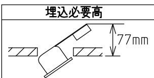
傾斜天井使用可能 (55°まで)
