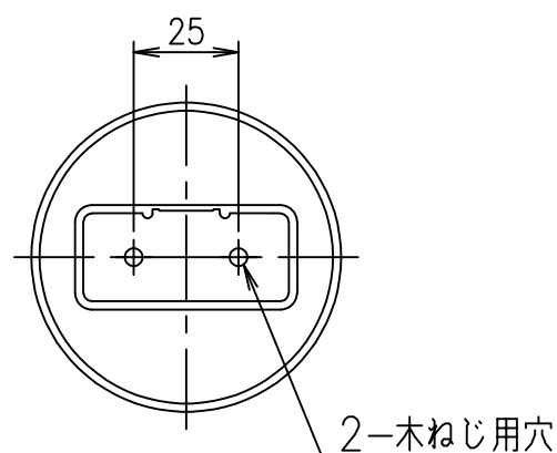
取付部詳細
