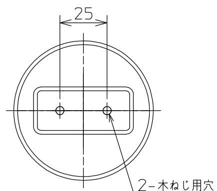
取付部詳細
