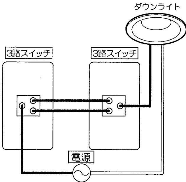
[3路スイッチ配線]
