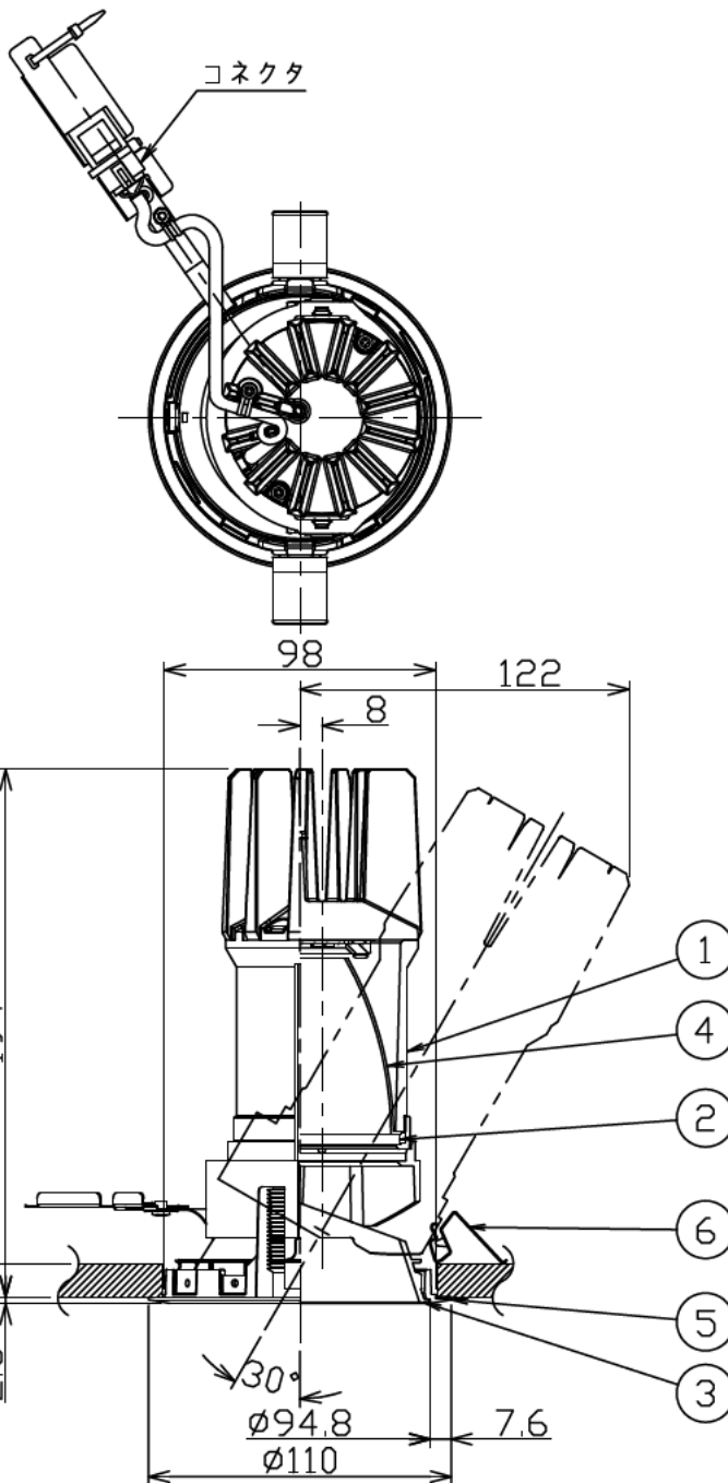
埋込穴寸法
