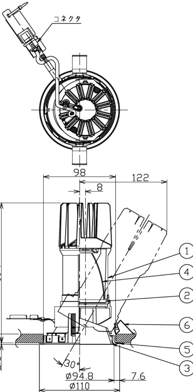
埋込穴寸法
