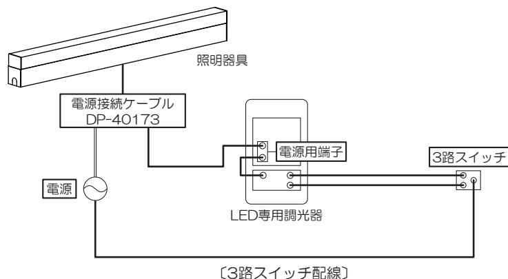
〔3路スイッチ配線〕
