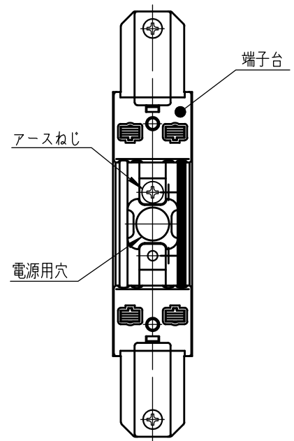
端子台詳細
