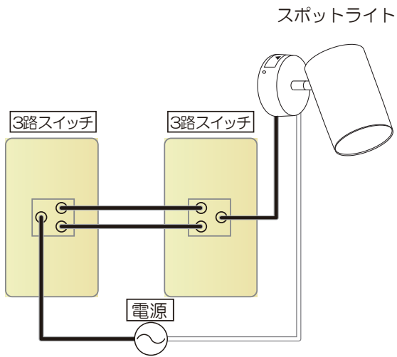
[3路スイッチ配線]
