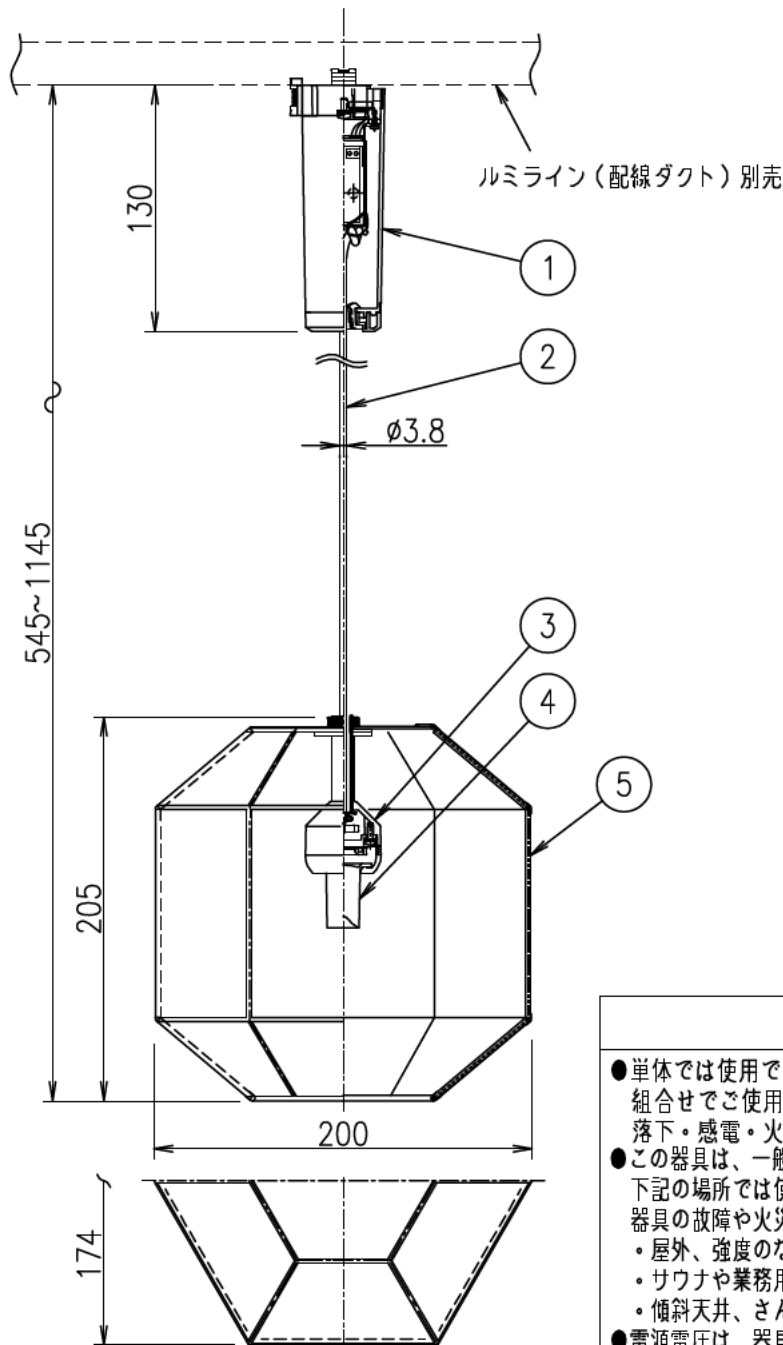
取付詳細図
