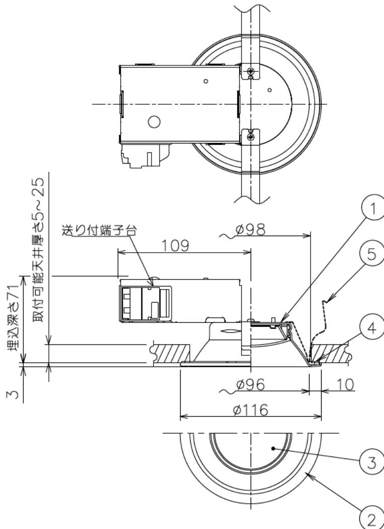
埋込穴寸法
