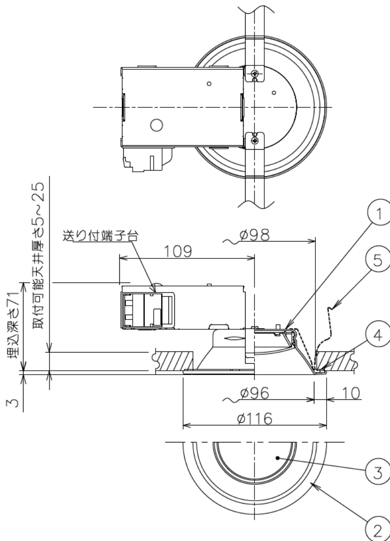
埋込穴寸法
