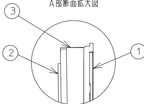
A部断面拡大図
