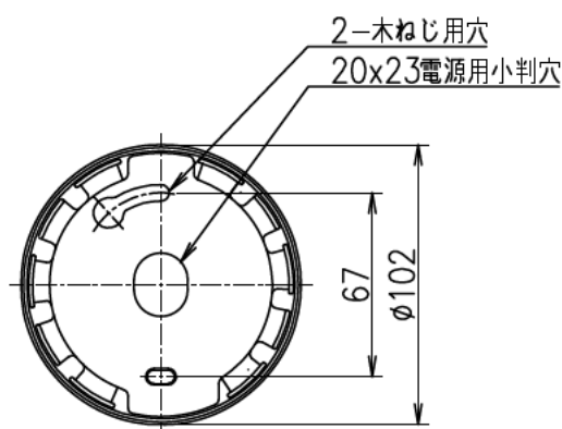
取付詳細図
