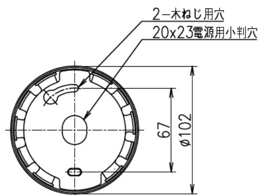
取付詳細図
