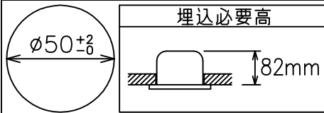
埋込穴寸法
