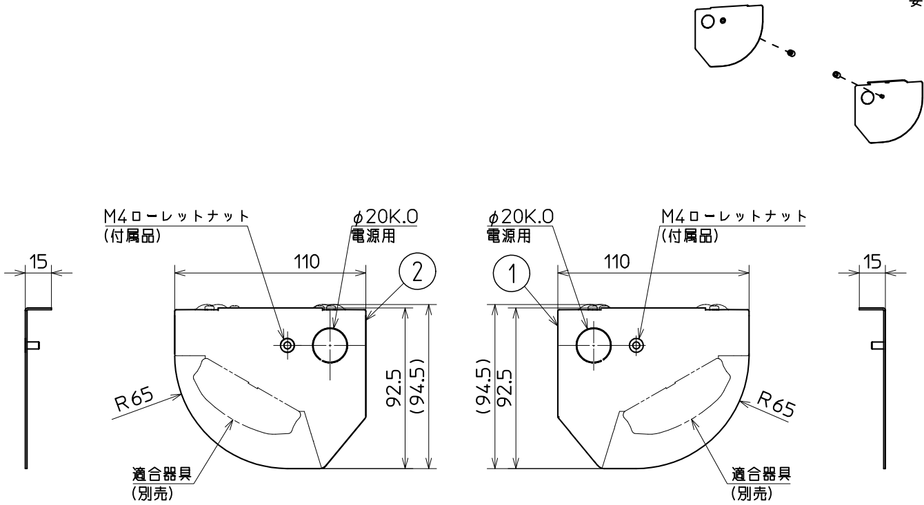
器具取付け状態
