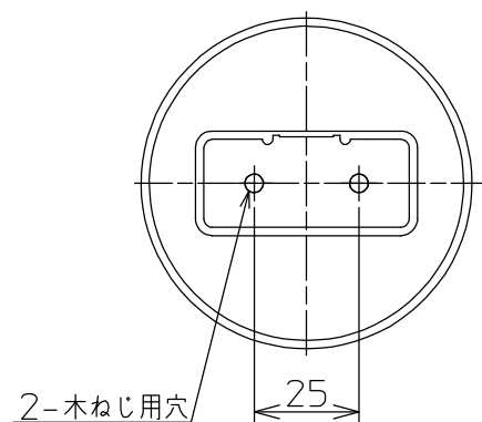
取付部詳細
