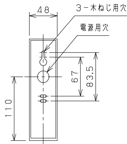
取付部
