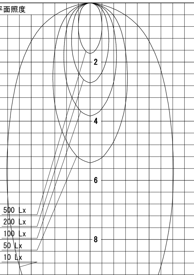
配光曲線
