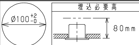
埋込穴寸法
