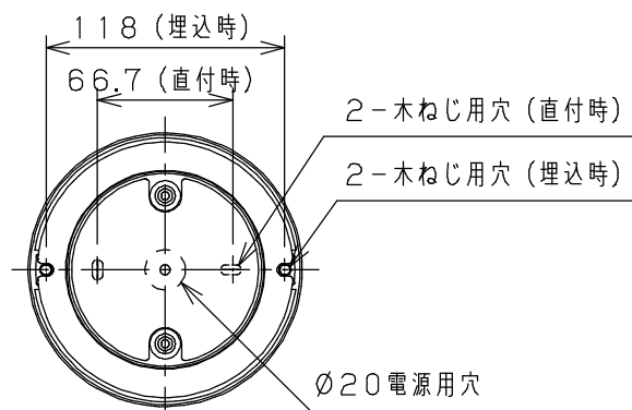
取付部詳細
