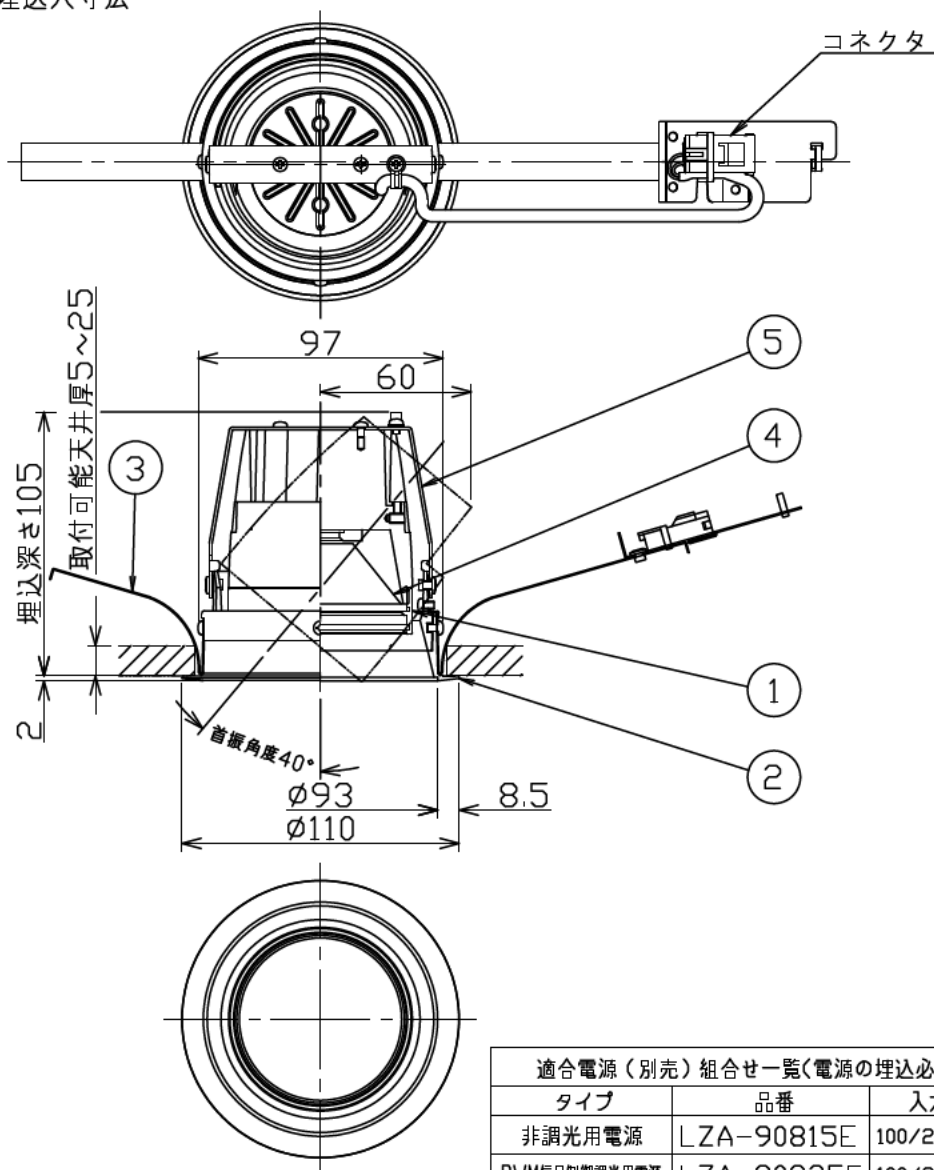
埋込穴寸法
