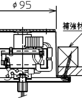
天井埋込時
