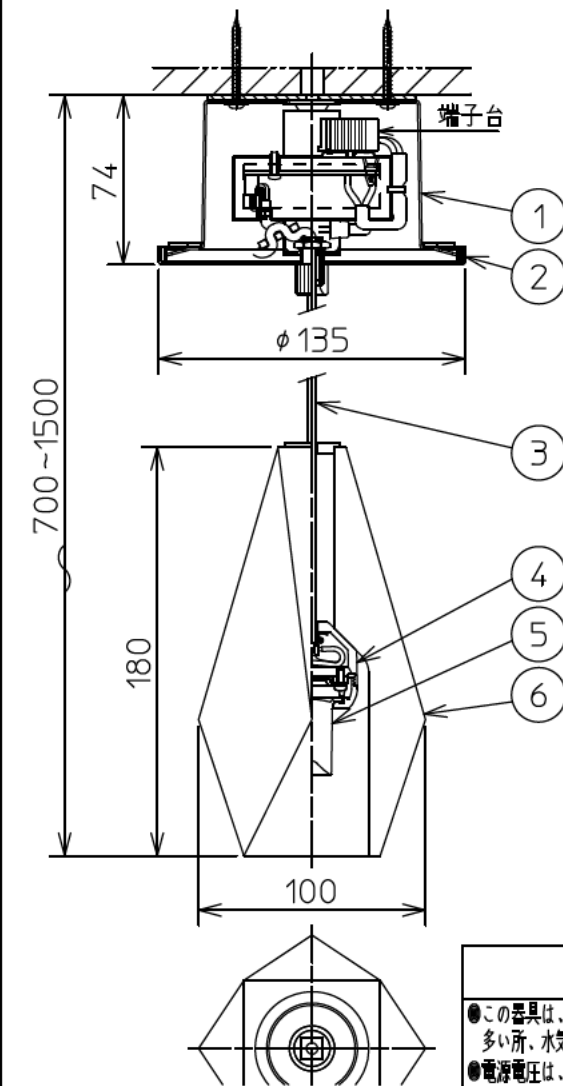
天井直付時
