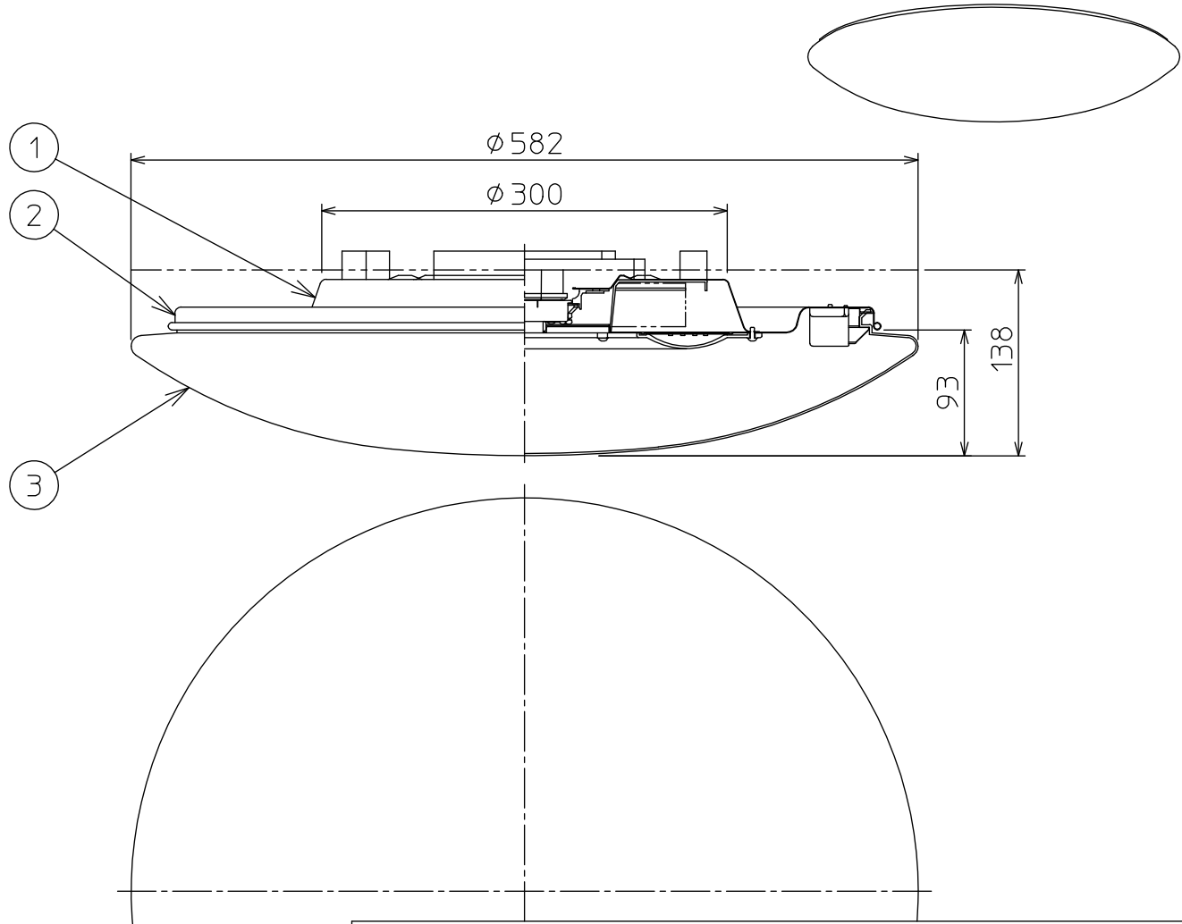
姿図
