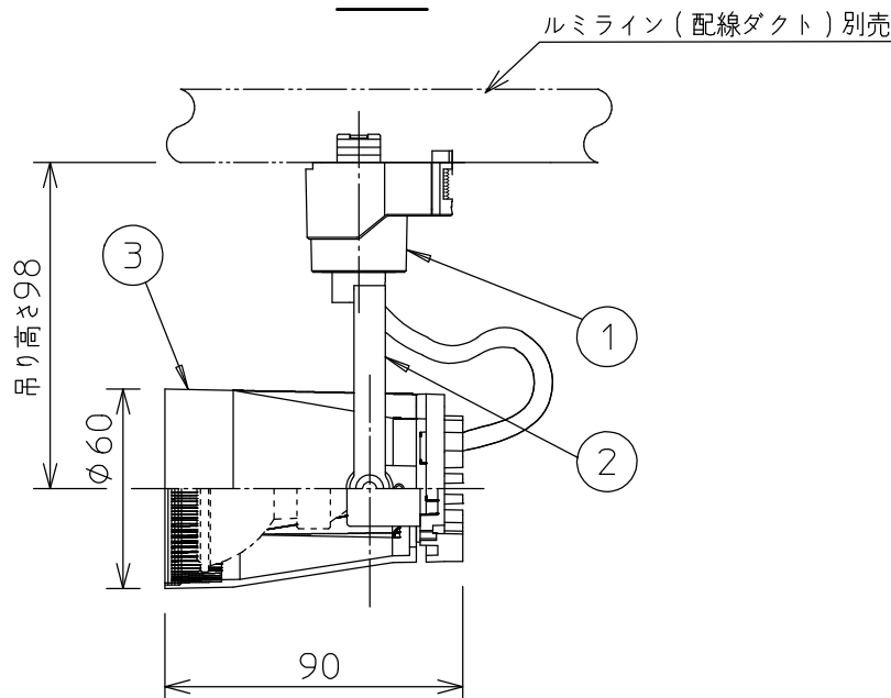
取付部
