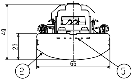
側面詳細図
