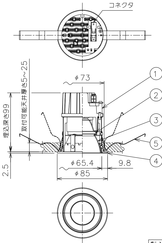
埋込穴寸法
