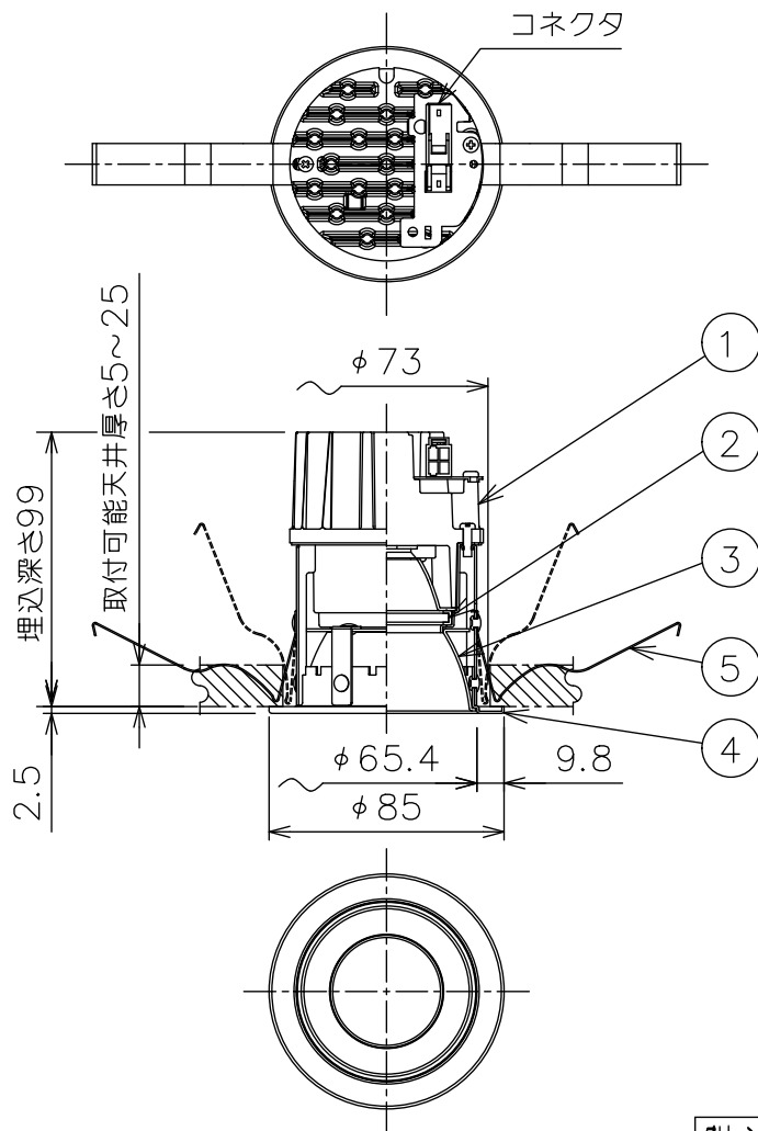
埋込穴寸法
