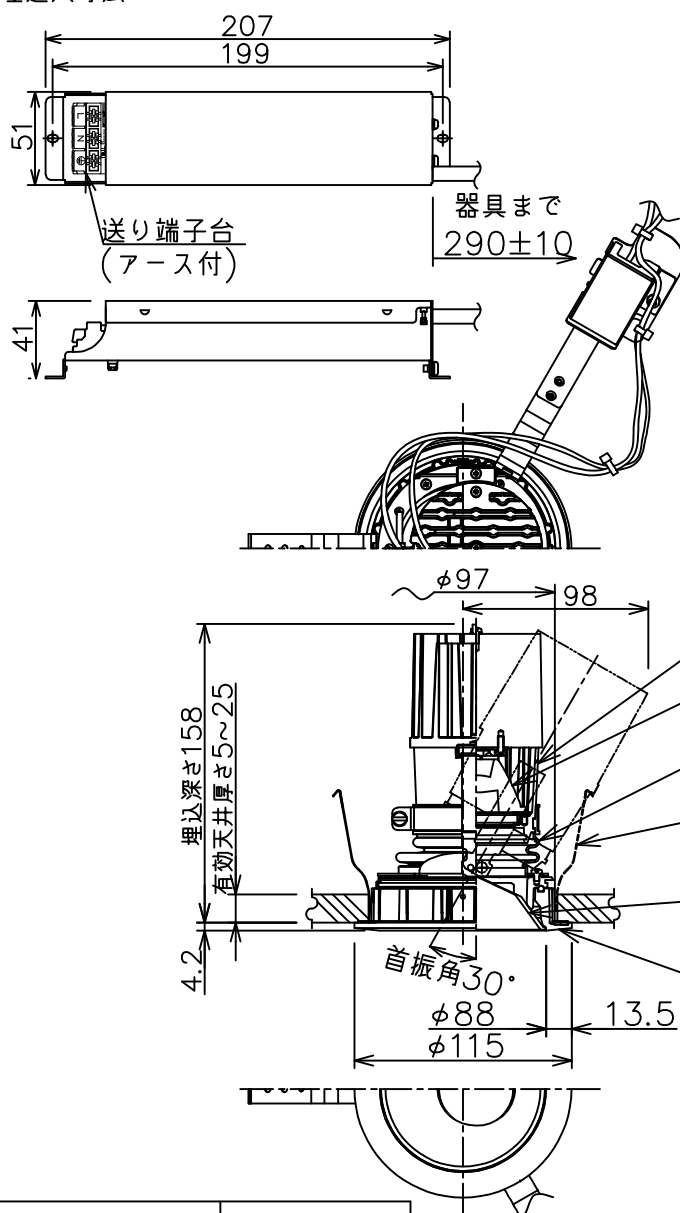
埋込穴寸法
