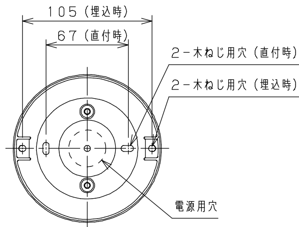
取付部詳細
