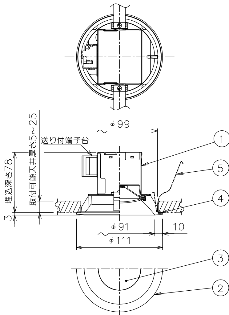
埋込穴寸法
