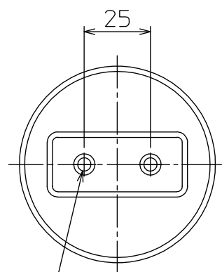
取付部詳細
