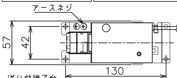
埋认穴寸法
