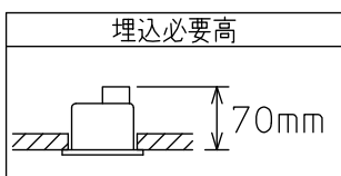
傾斜天井使用可能(55°まで) 端子台を必ず上側に 向けてください。
