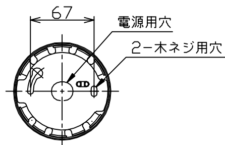
取付部詳細
