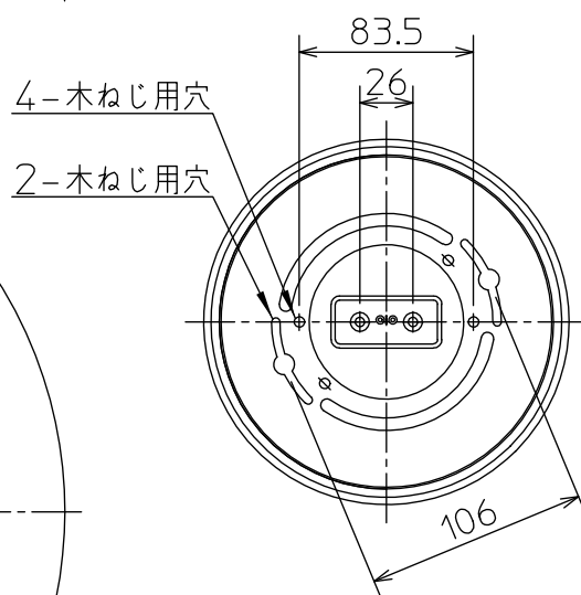
取付部詳細
