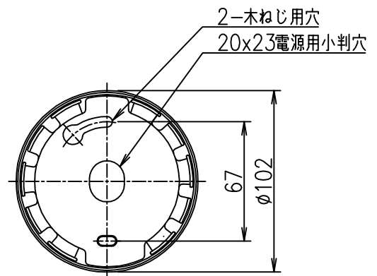
取付詳細図
