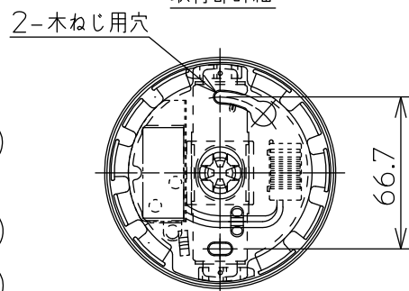
取付部詳細
