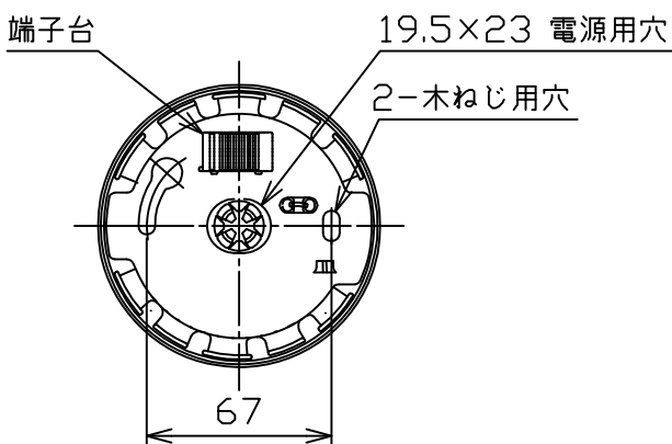
取付部詳細
