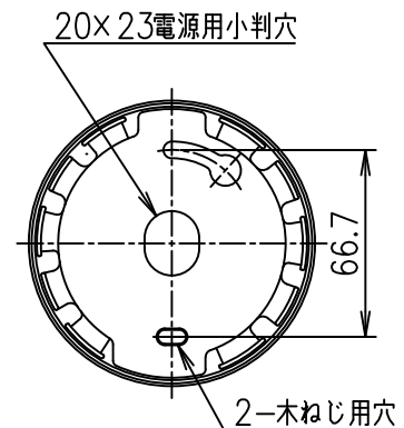
取付部詳細
