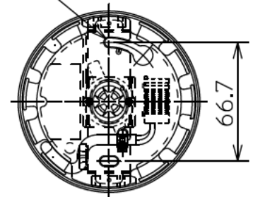
取付部詳細
