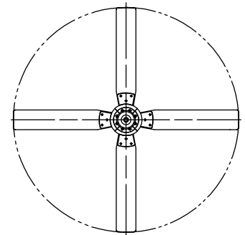
羽根配置図
