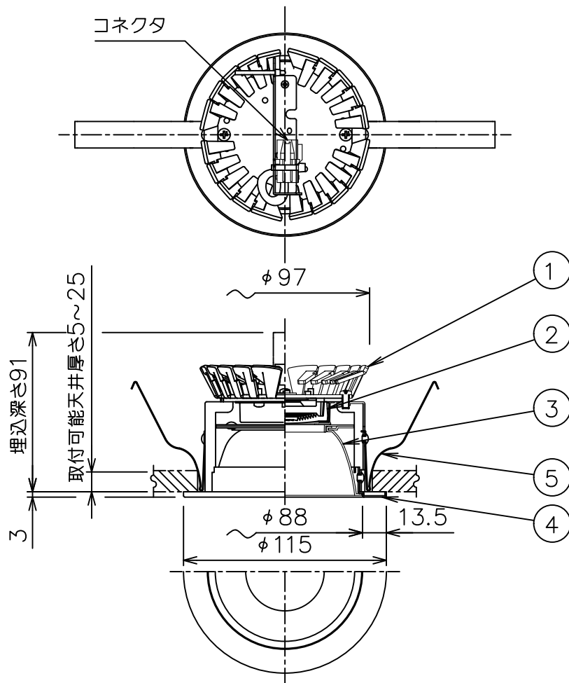
埋込穴寸法
