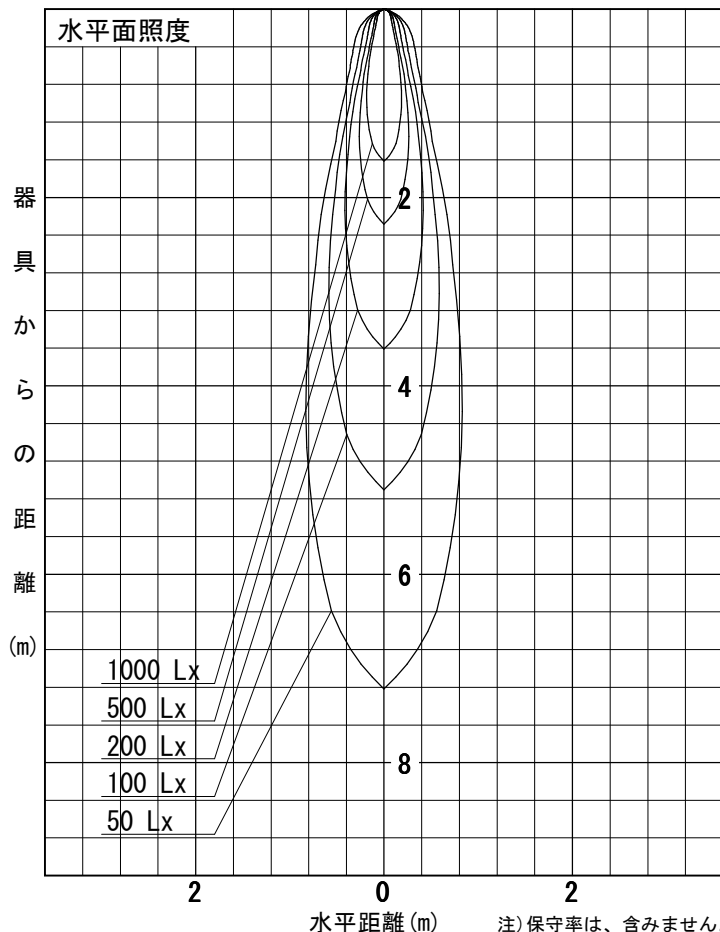
配光曲線
