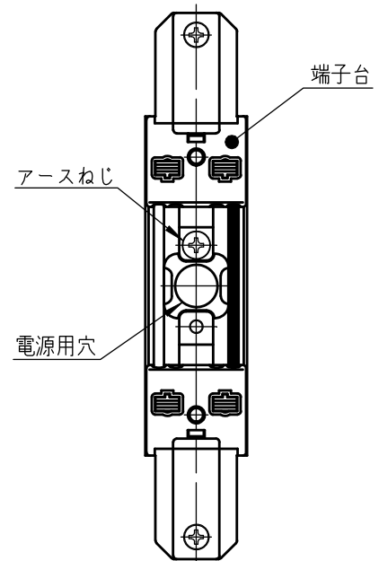
端子台詳細
