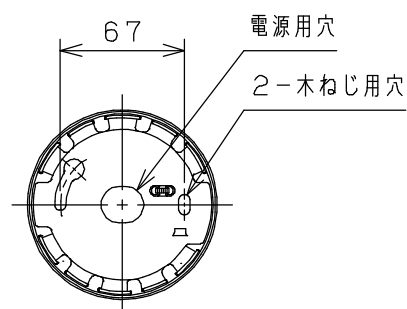
取付部詳細
