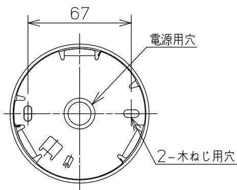
取付部
