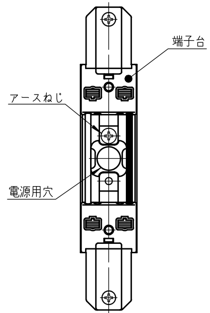
端子台詳細
