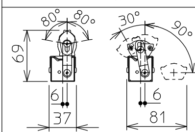
灯具可動範囲
