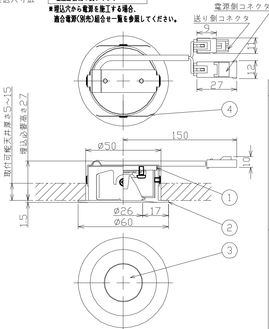
埋込穴寸法
